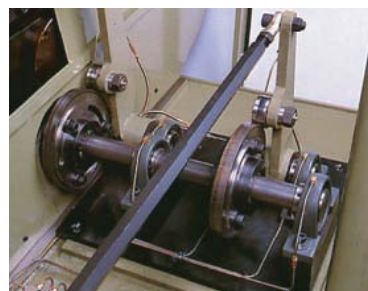
▲2スターターカム(25R型のみ)
